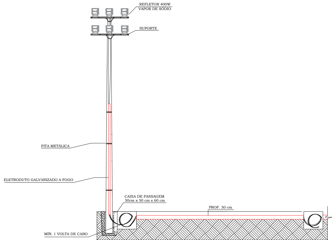
DETALHE POSTE COM REFLETORES E CAIXA DE PASSAGEM
