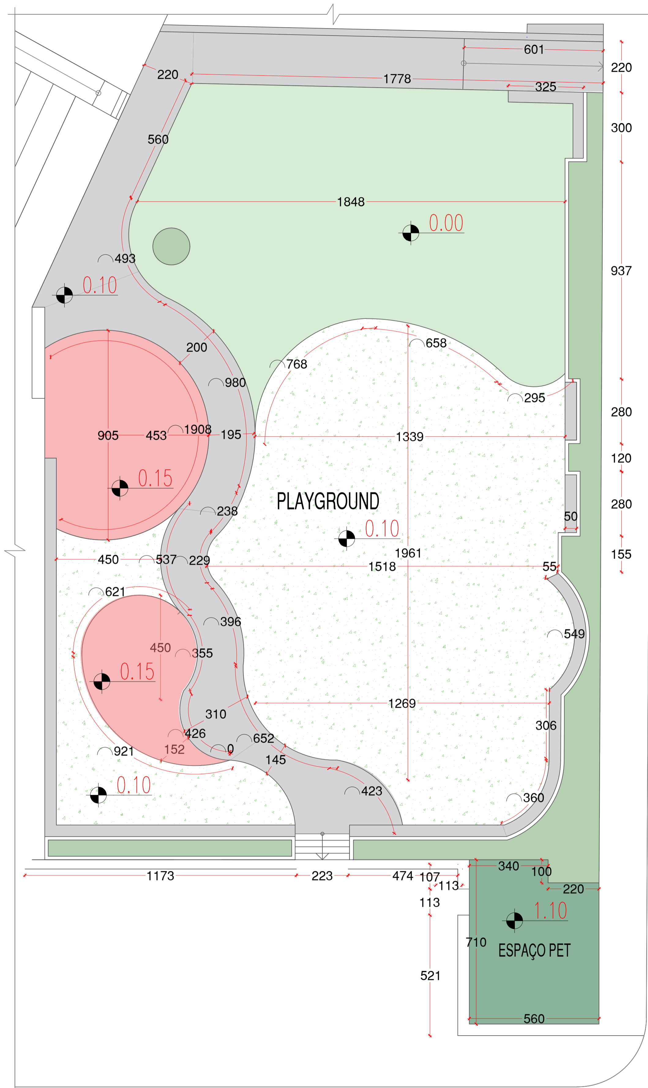
01 Planta baixa - Projeto Novo Playground e Espaço Pet ESCALA: 1/100
