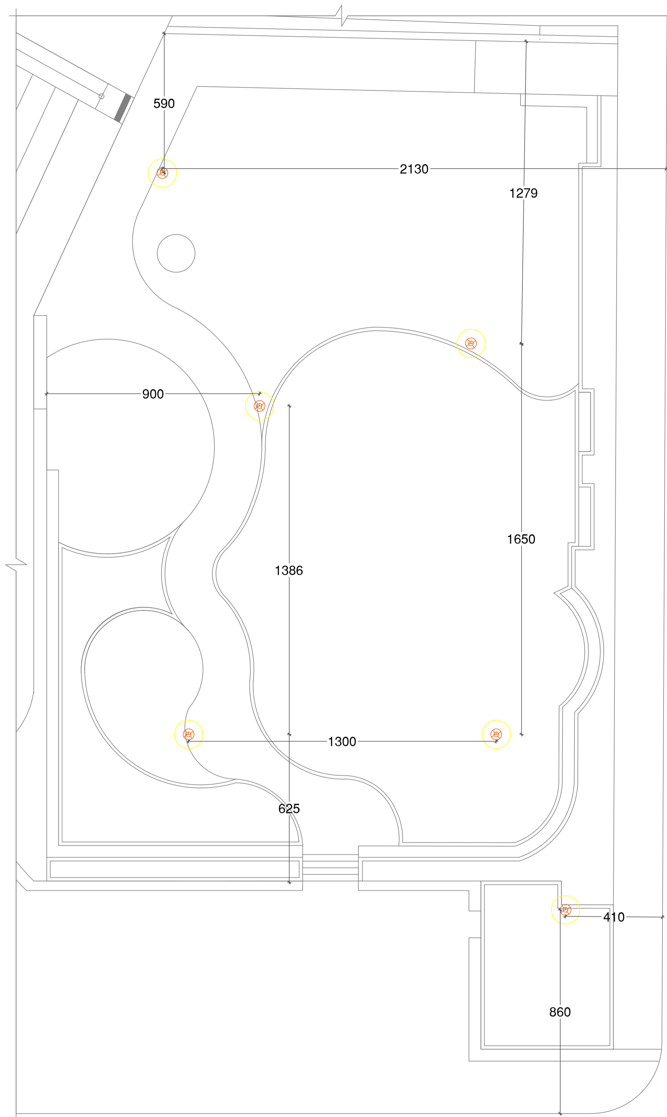
01 Planta de Locação dos Postes ESCALA: 1/100
