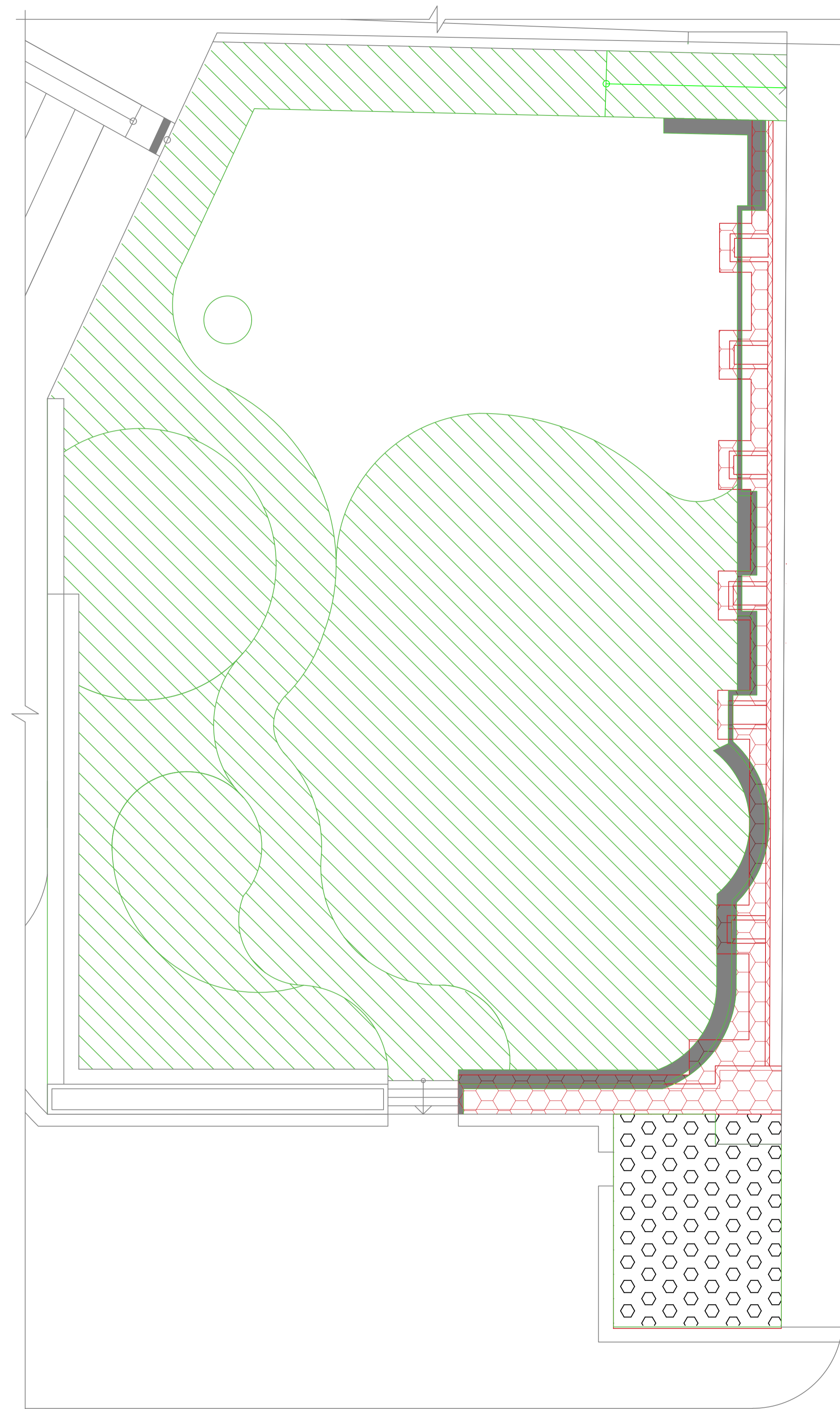
02 Planta - Demolição/Construção ESCALA: 1/100
