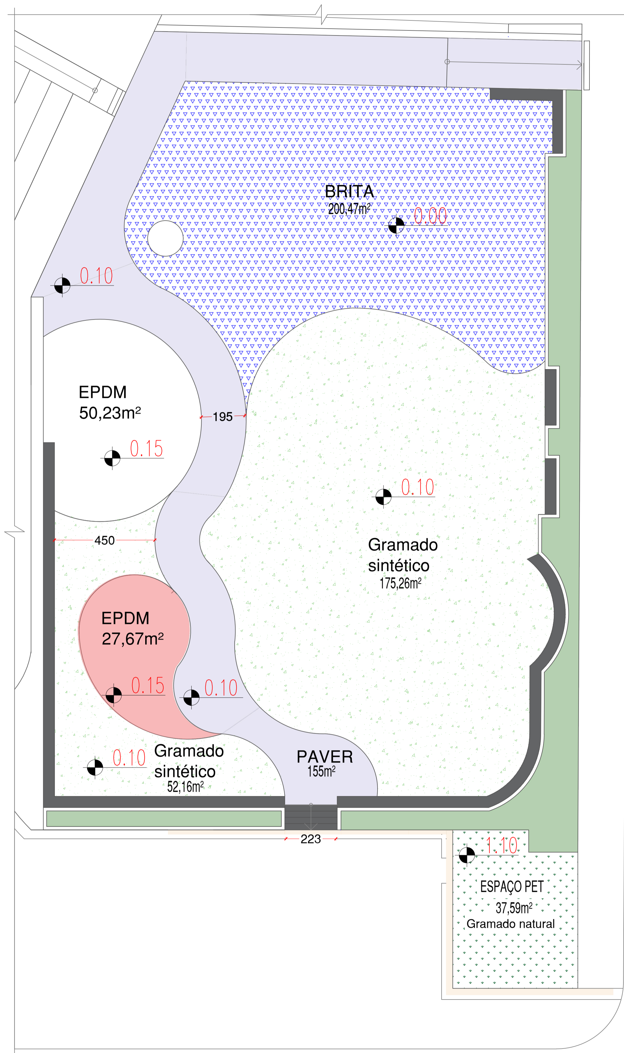
01 Planta de Tipos de Pavimentação ESCALA: 1/100
