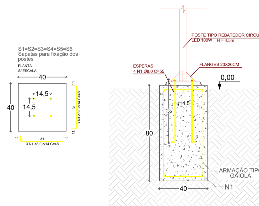
04 Detalhamentos ESCALA: S/ Escala
